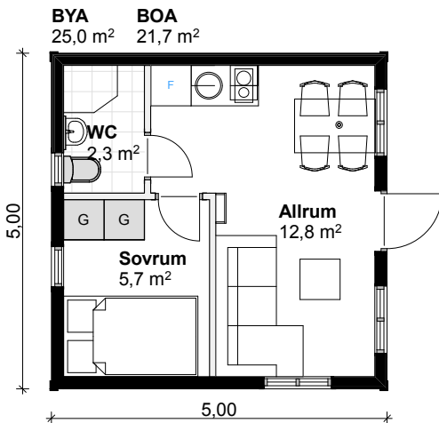
1. Våning 1 1:100
