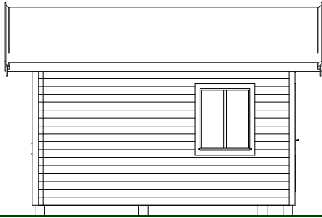
A1 Fasad A1 1:100
