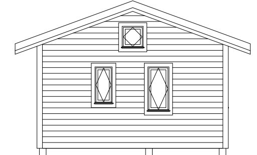
A4 Fasad A4 1:100
