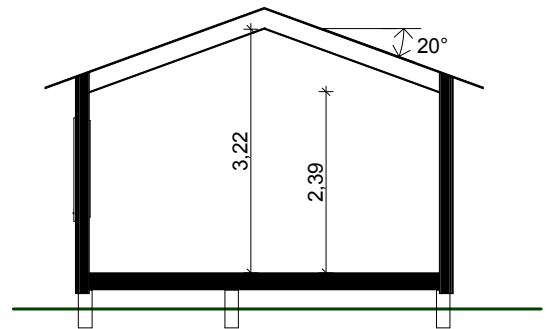
S2 Allrum 1:100
